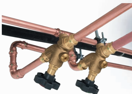
V systému: kulové kohouty s lisovaným spojem.
